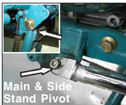
Lever Pivot
